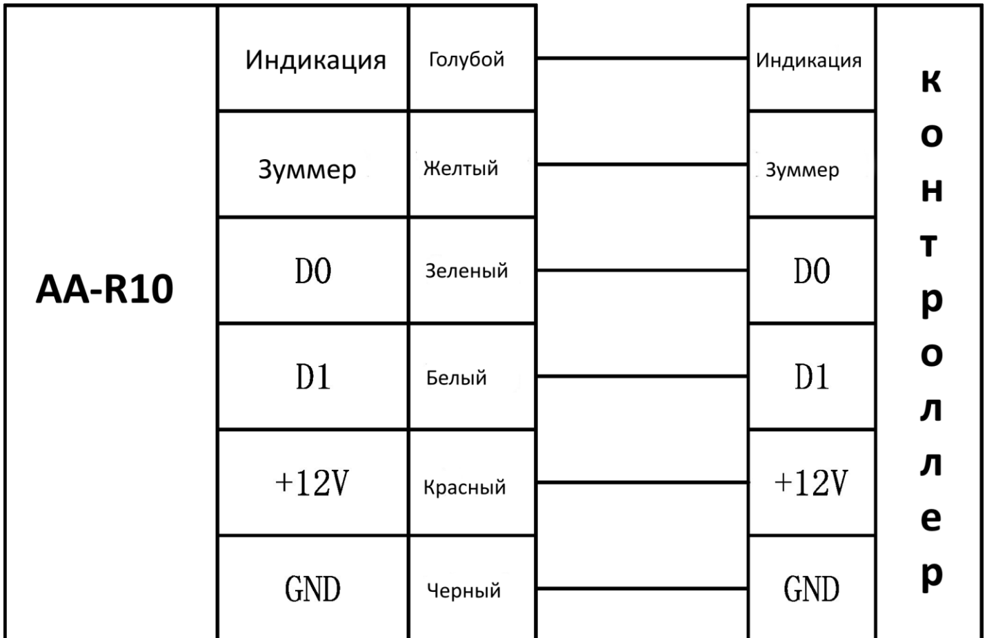
Схема подключения Аxiom AA-R10
