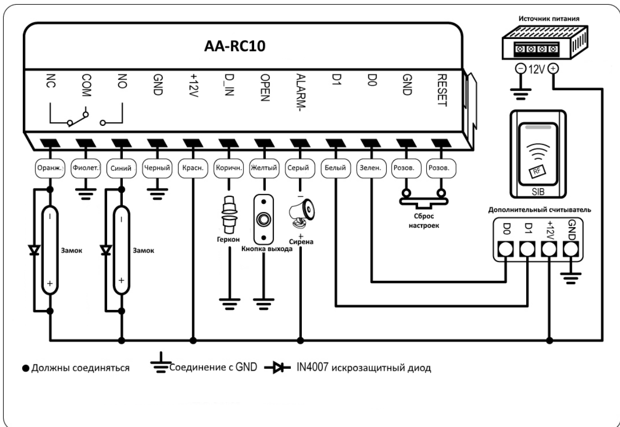
Схема подключения Axiom AA-RC10
