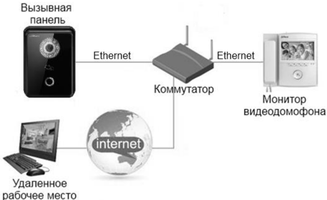
Схема подключения DHI-VT06210B
