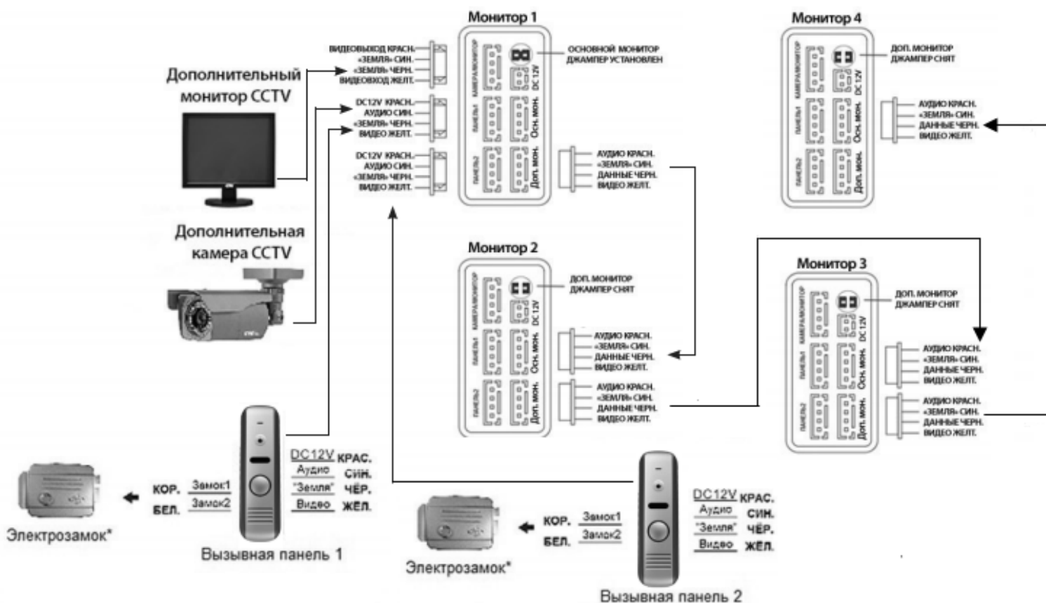
Схема подключения AA-VDP702SW
