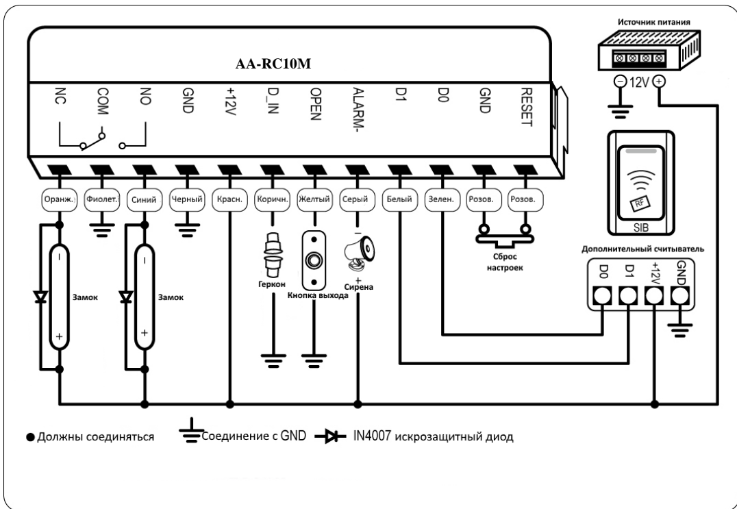
Рис. 1 Схема подключения для одной двери с использованием стандартного источника питания
