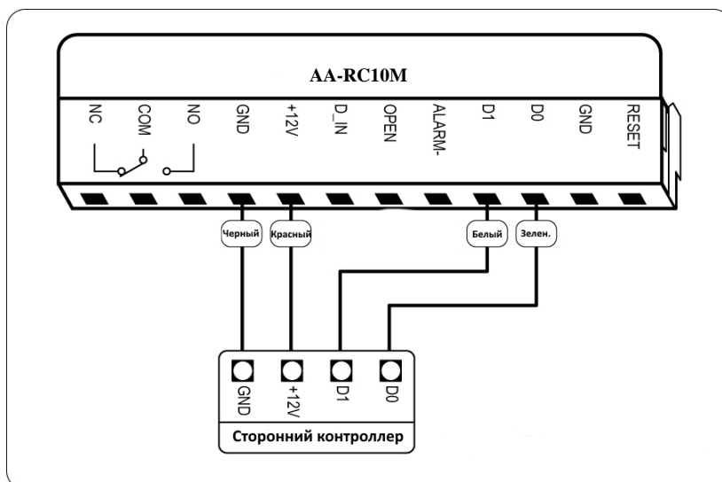
Рис. 3 Схема подключение AA-RC10M в качестве считывателя
